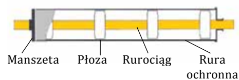
Przekrój rurociągu po ułożeniu.
